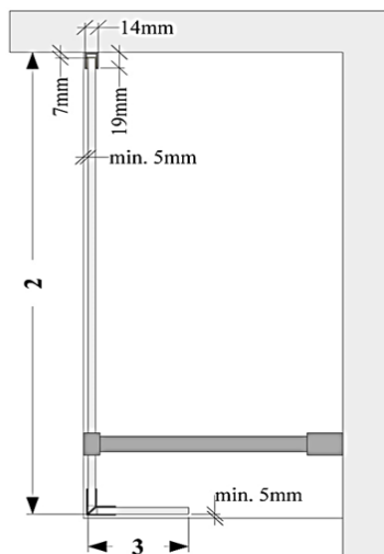
Bovenaanzicht
