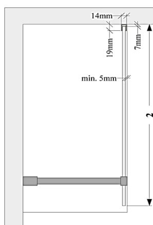
Bovenaanzicht
