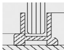
Profilé sur bac de douche Très bonne étanchéité
