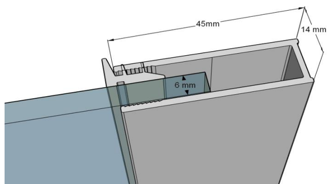
muurprofiel / profilé mural
