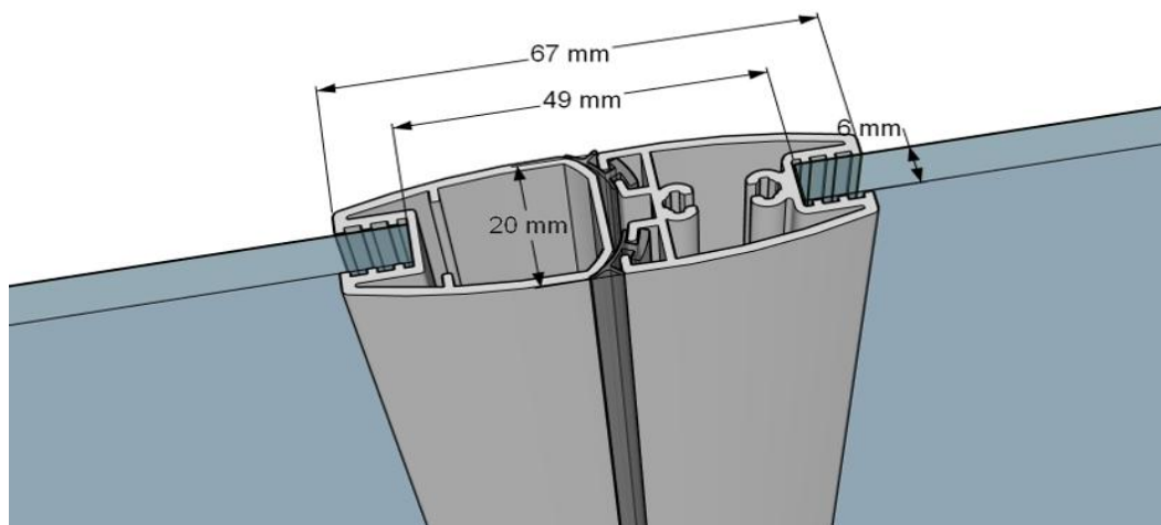
scharnierprofiel / profilé charnière
