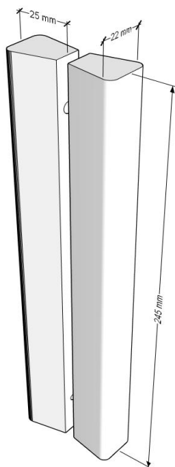
Greep / Poignée
