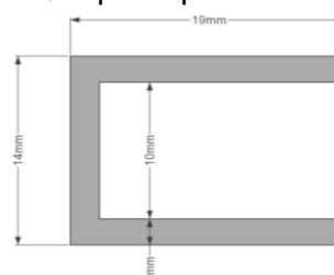
Muurprofiel/profilé mural
